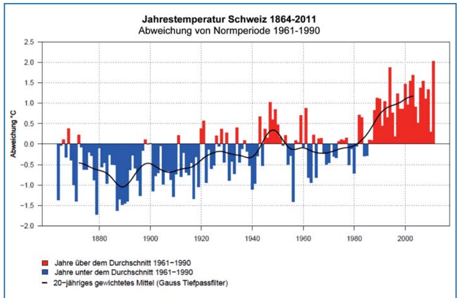
Bild 1. Abweichung der Jahrestemperatur in der Schweiz gegenüber der Klima-Normperiode 1961–1990. Die schwarze Kurve zeigt den Temperaturverlauf gemittelt über 20 Jahre. Das Jahr 2011 (letzter Eintrag) zeigt einen Temperaturüberschuss von +2°C und ist damit das wärmste Jahr seit Messbeginn (Quelle: MeteoSchweiz, 2012).
